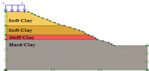
Gambar 2. Pemodelan Lereng Alami pada Program Plaxis
