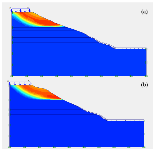
Gambar 5. Output lereng alami (a) Potongan 2-2 dan (b) Potongan 3-3
