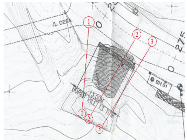
Gambar 4. Peta Topografi (PU Bina Marga, 2015)
